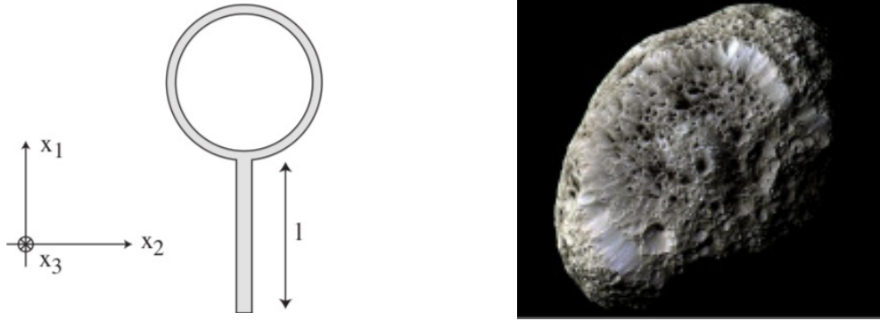
Figure 2: Gauche : Modélisation d'une raquette de tennis. Droite : Photographie d'Hyperion. Source https://www.le-systeme-solaire.net/hyperion.html
